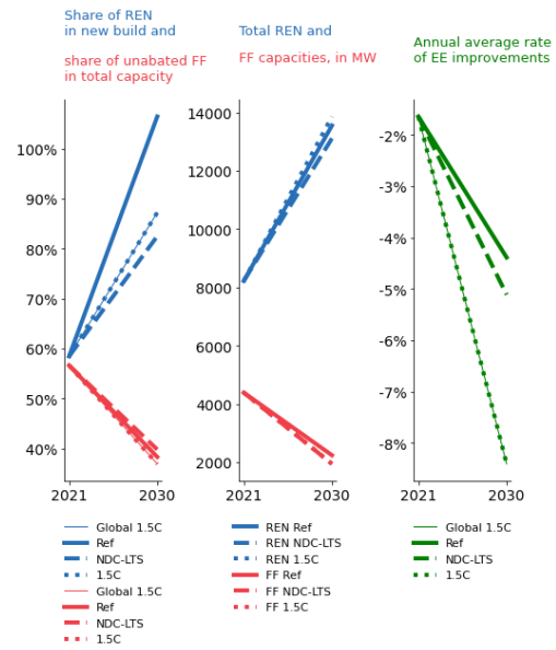
Decarbonisation indicators
