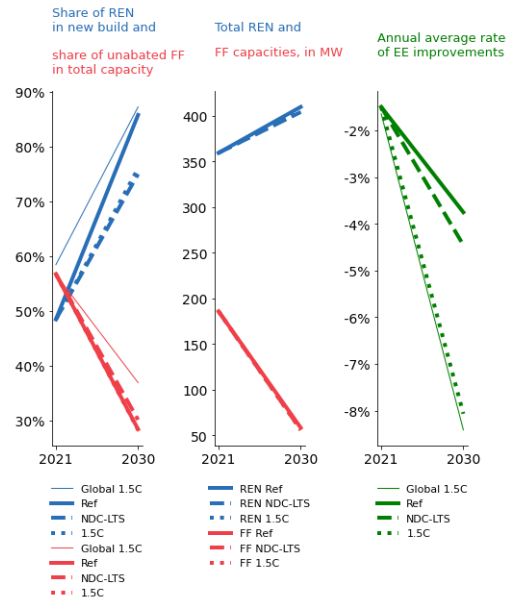
Decarbonisation indicators
