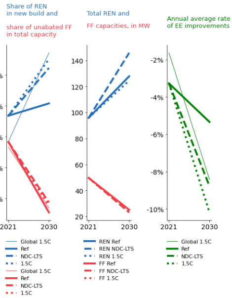
Decarbonisation indicators
