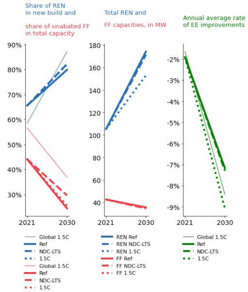
Decarbonisation indicators
