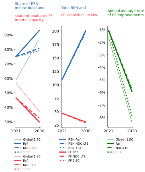
Decarbonisation indicators
