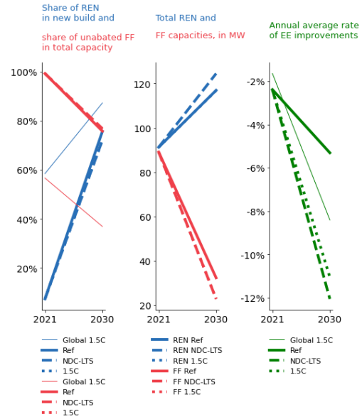
Decarbonisation indicators
