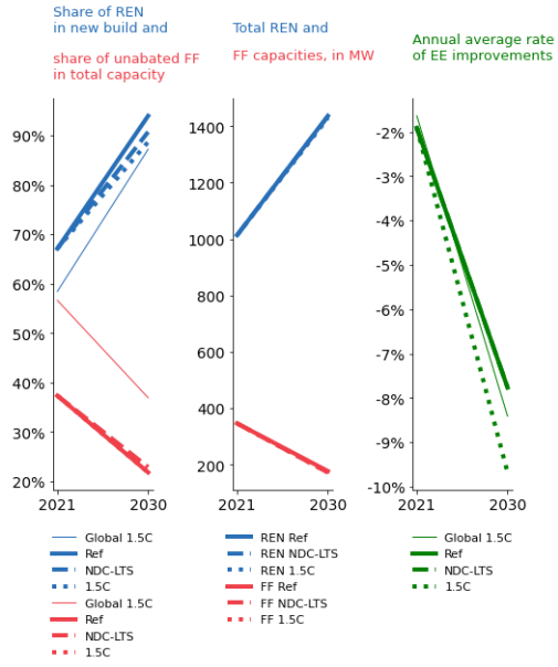
Decarbonisation indicators
