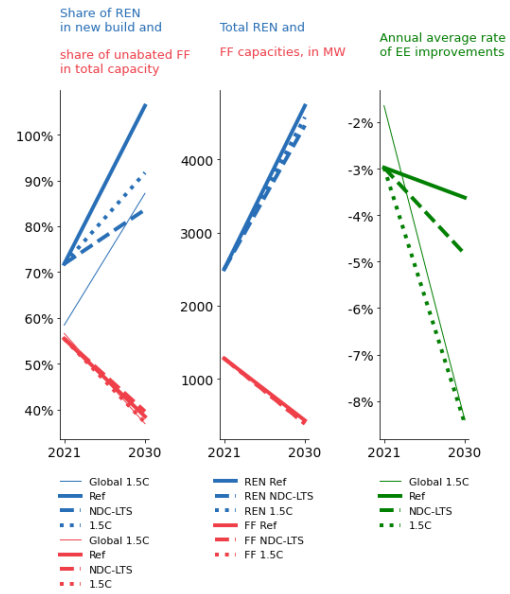
Decarbonisation indicators
