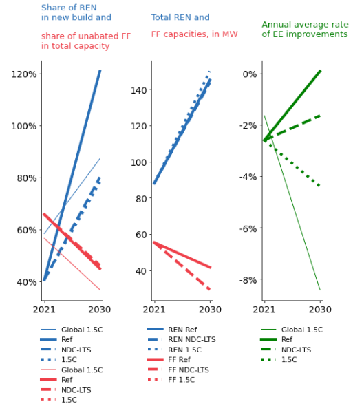
Decarbonisation indicators
